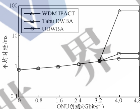
图 5 高优先级数据帧平均时延
