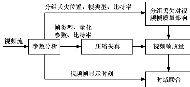
图 7 只分析视频头的比特流层评价模型
