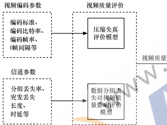
图2 网络参数规划模型
